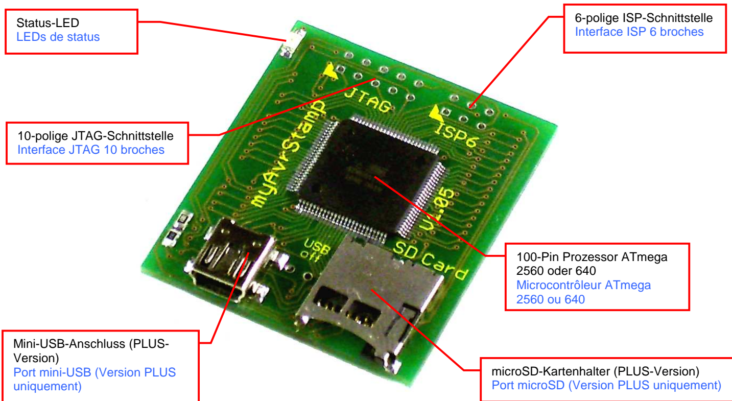
myAVR Stamp Vorderseite / myAVR Stamp recto
